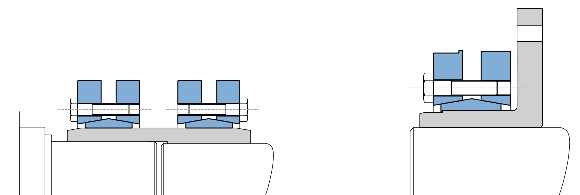
Utilização do modelo TLK 603 como união entre veios de diferentes tamanhos
