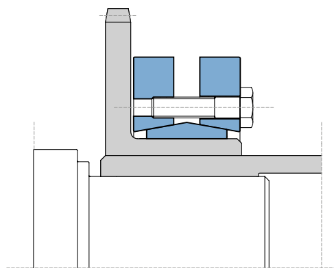
Fixação simultânea de uma roda dentada e de um veio oco.
