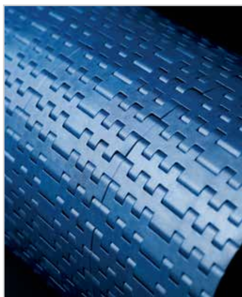
Cadena MatTop de la serie 395 de Rexnord (vista superior)
