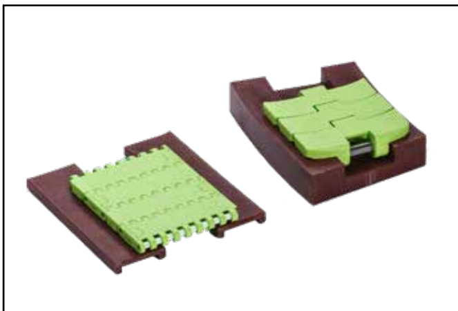
Cadena Dry-PT de Rexnord junto con las guías de deslizamiento ULF de Rexnord
