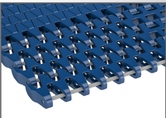
Módulo final del diseño mejorado de la cadena MatTop de la Serie 1275-1285 de Rexnord
