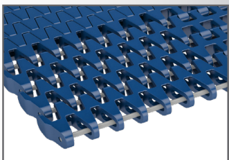
Module d'extrémité amélioré Série de chaînes Rexnord MatTop 1275-1285
