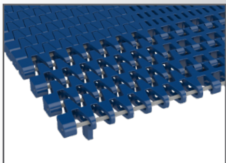
Module d'extrémité d'origine Série de chaînes Rexnord MatTop 1275-1285
