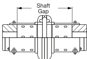
Ambos núcleos montados hacia afuera
