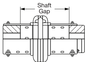
Un núcleo montado hacia afuera Un núcleo montado hacia adentro
